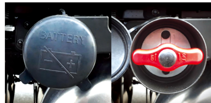
배터리 컷오프 스위치 장기 주차 시 배터리 방전 방지 및 편의성 증대
